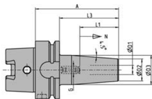
Aufnahme HSK-A63 für Schaftfräser / Schrumpffutter Chuck HSK-A63 for end milling cutter / Shrink Chucks
