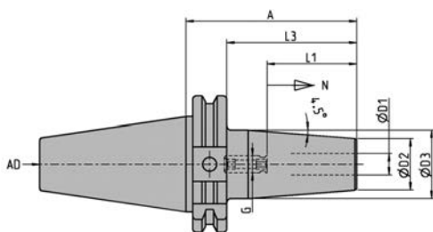
Aufnahme AD40 für Schaftfräser / Schrumpffutter Chuck AD40 for end milling cutter / Shrink Chucks
